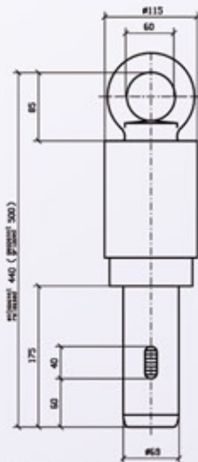
Maßzeichnung AL 70/76
